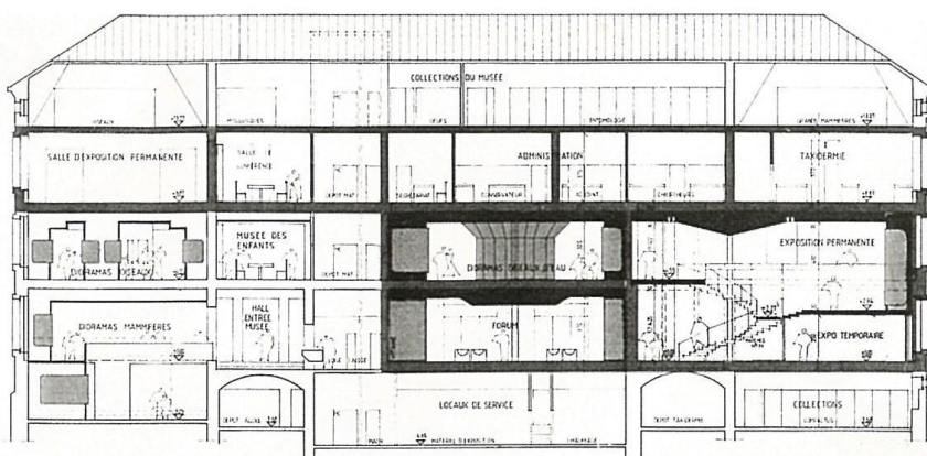
COUPE LONGITUDINALE
